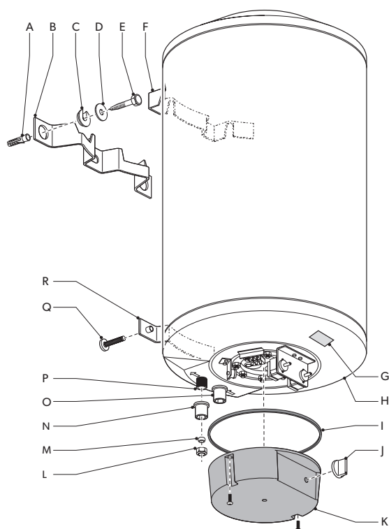
Figuur 1 Hoofdcomponenten
