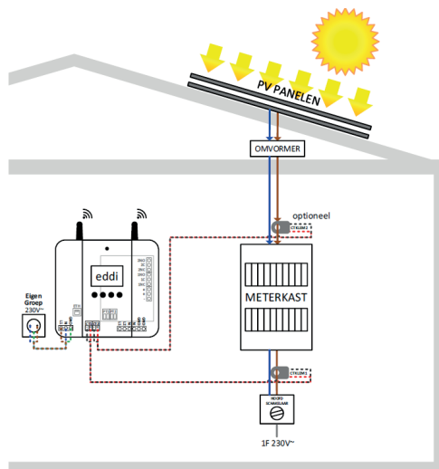
1 fase voeding + 2 CT-klemmen bedraad
