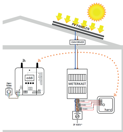
3 fase voeding + 3 CT-klemmen bedraad
