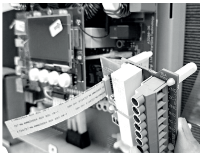
Figuur 2 Plaats het losse relais- en sensorbord op het moederbord
