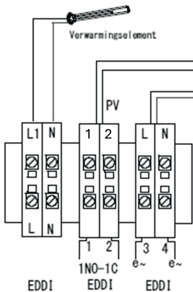
Figuur 5 Aansluitblokken L, N en 1 t/m 4
