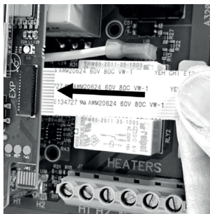
Figuur 2 Plaats het losse relais- en sensorbord op het moederbord
